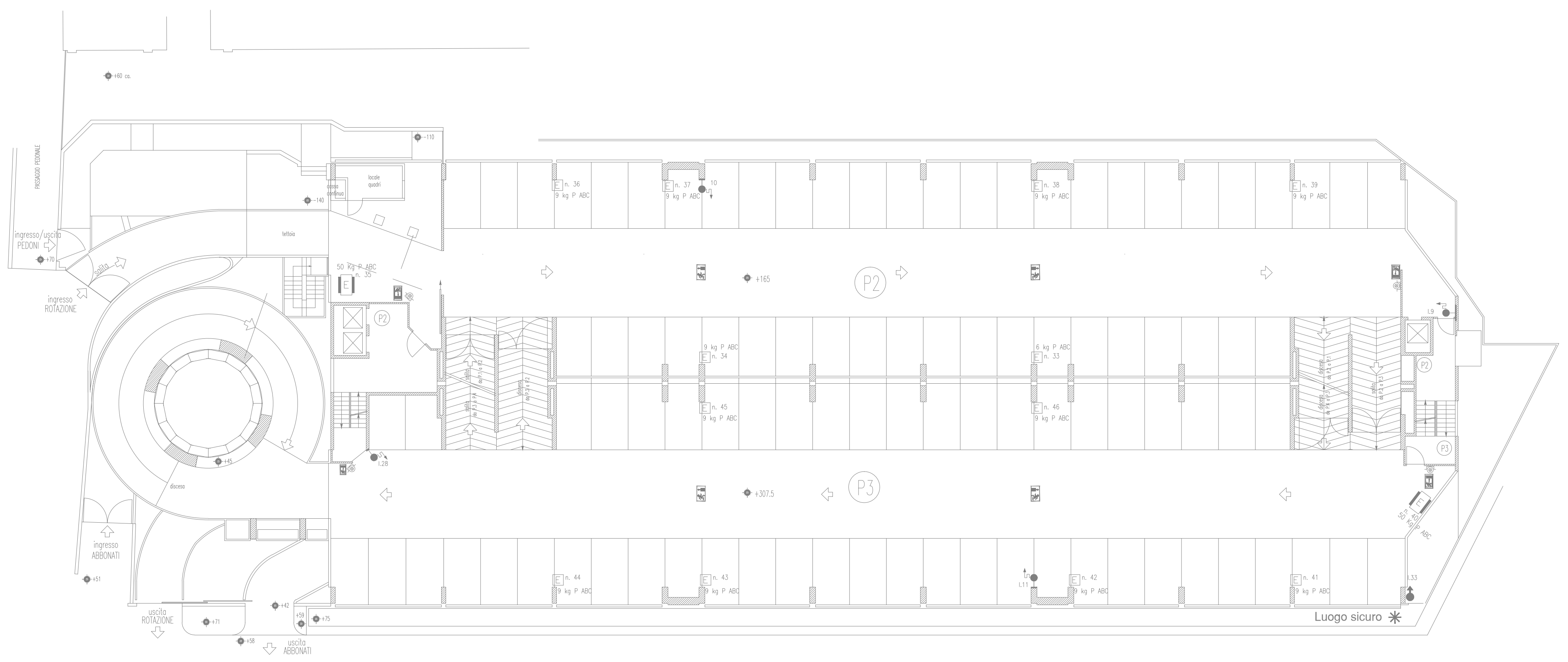
PIANTA PIANO TERRA - Livelli P.2, P.3
